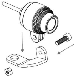
B. 前鏡鋁支架安裝
