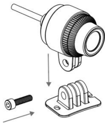
A. 前鏡黏貼座安裝
