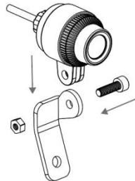
C. 後鏡鋁支架安裝
