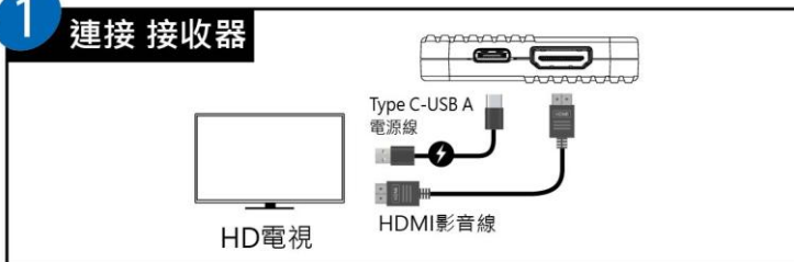
1.WTR-1500C 接收裝置 連接 顯示器設備
