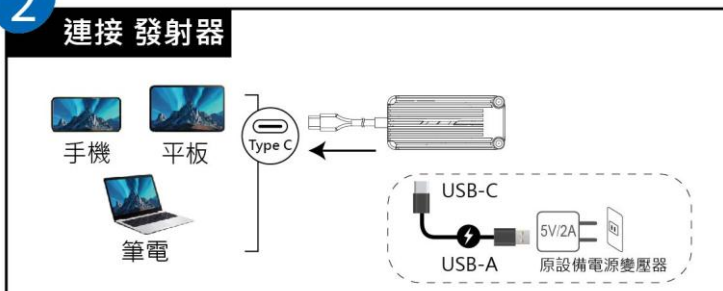
2.WTR-1500C發射裝置 連接 信號源設備
